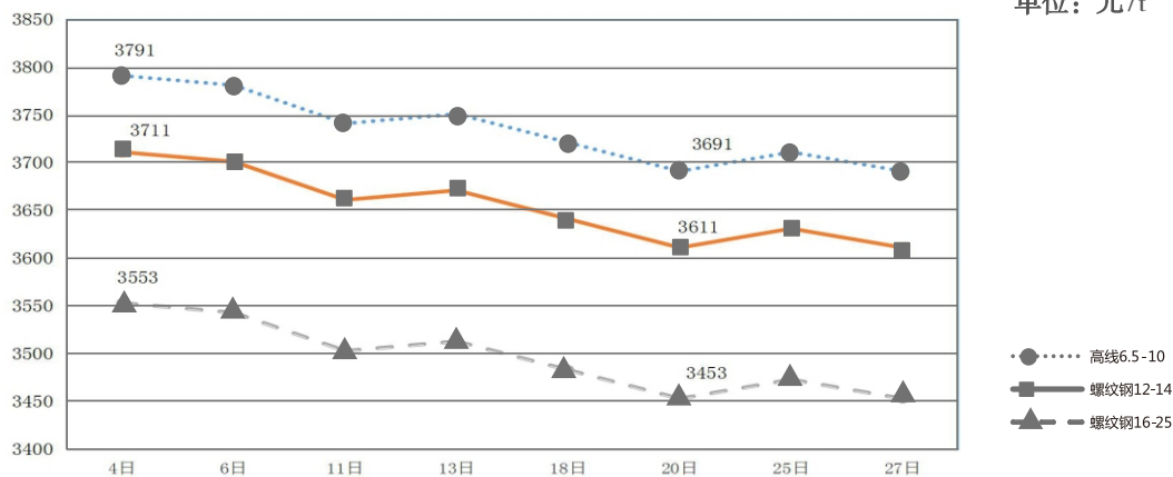
2025年3月中心城区主要钢材趋势图
