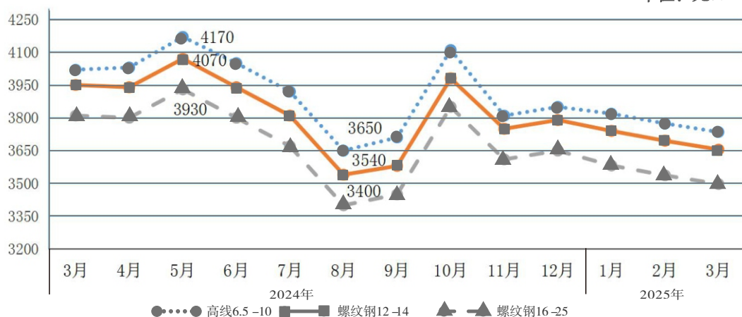
2024年3月—2025年3月中心城区主要钢材价格趋势图
