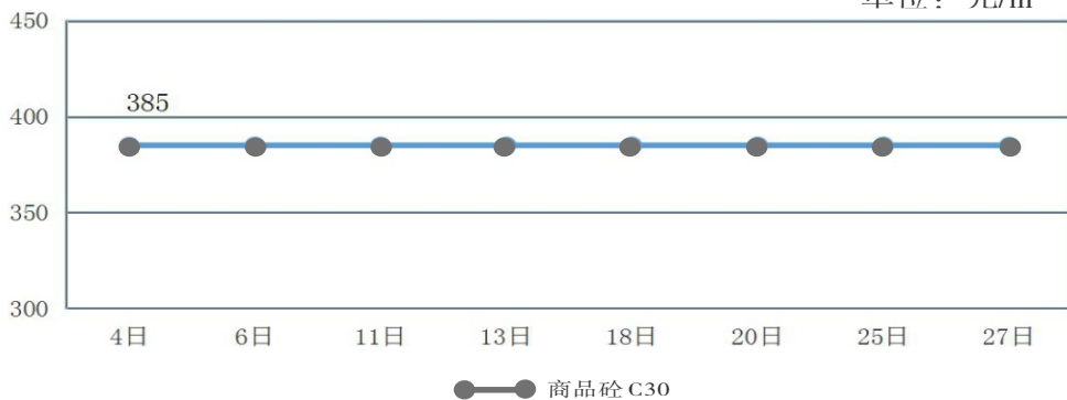
2025年3月中心城区商品砼C30 价格趋势图
