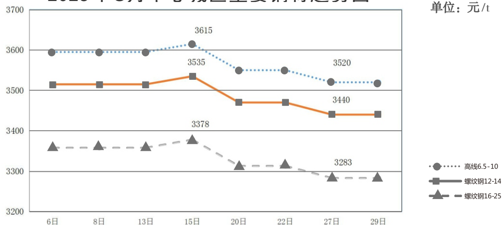
2025年5月中心城区主要钢材趋势图
