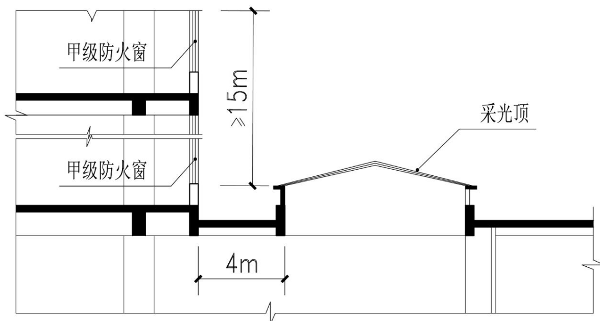
图3 主体建筑和采光顶开口示意图
